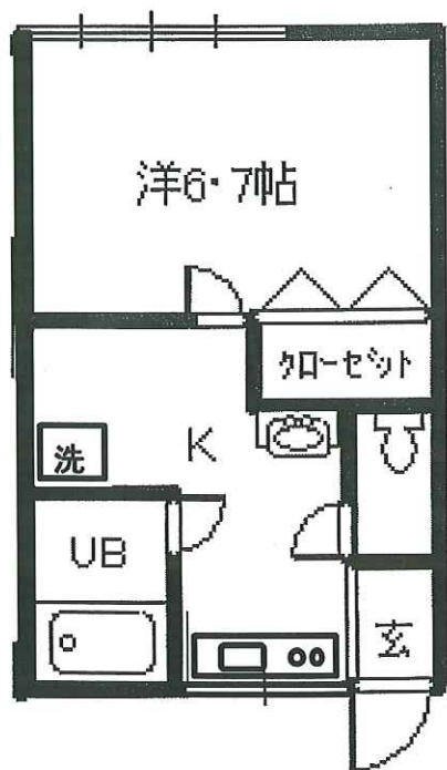
【間取図】
