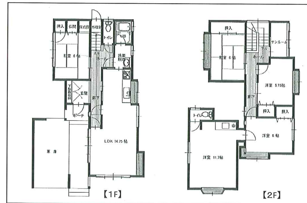
【間取図】
