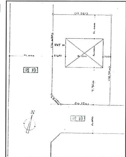
【配置図】
