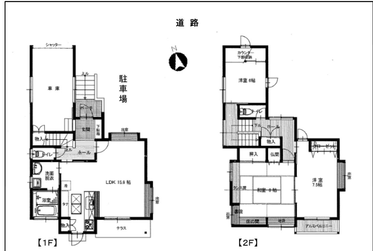
【間取り図】
