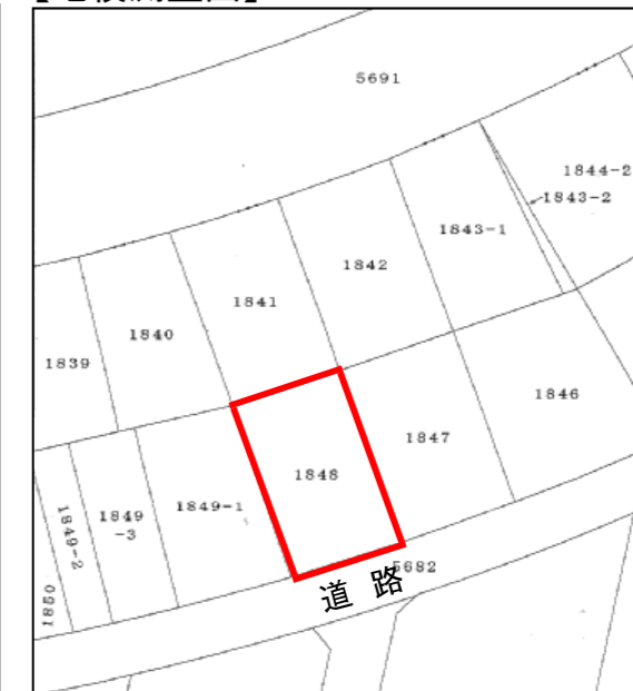
【地積測量図】
